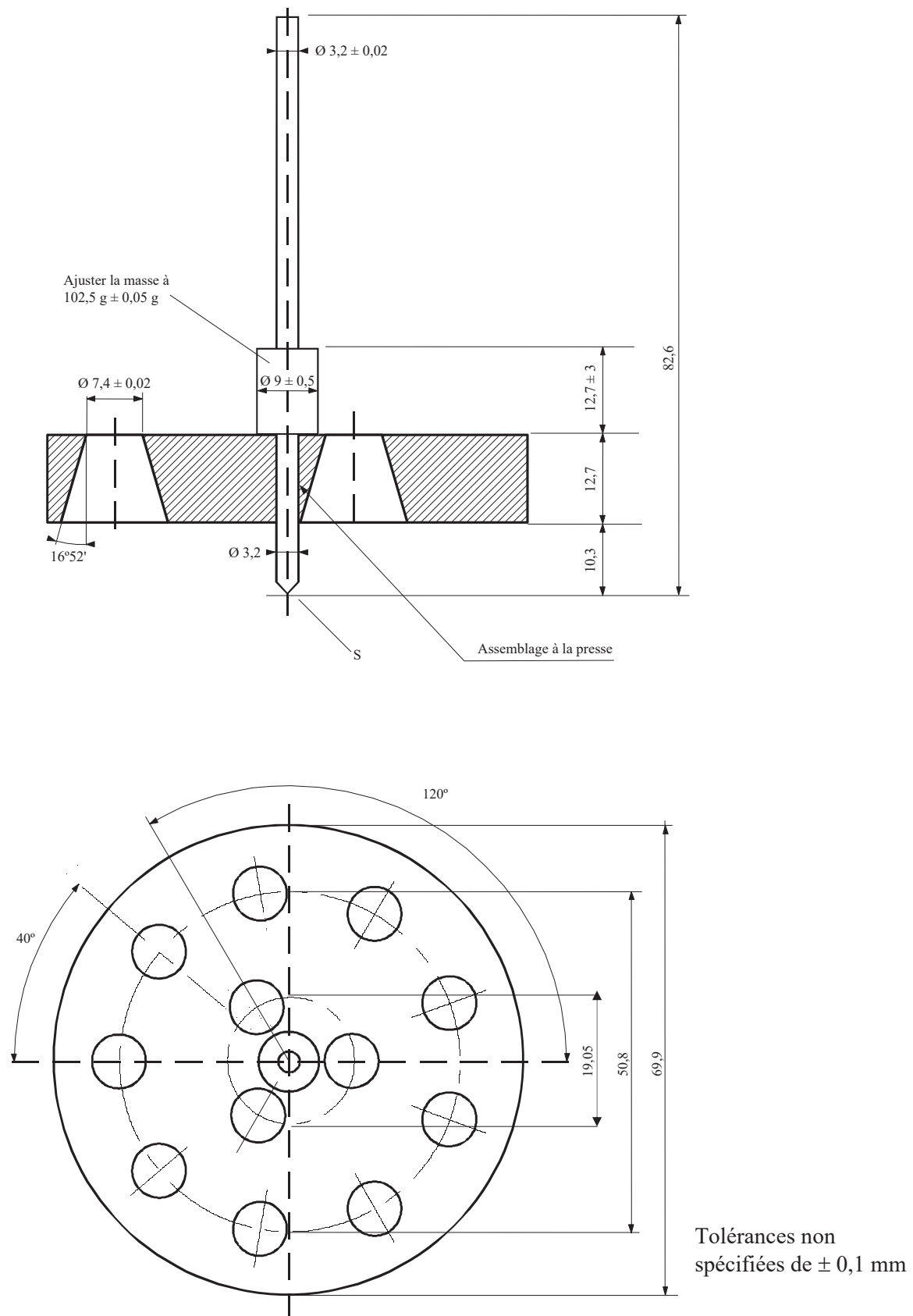
Figure 1 – Pénétromètre
